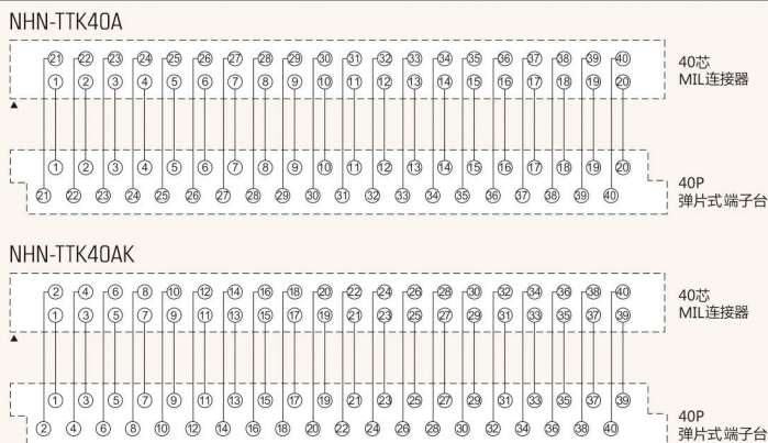
配线图 Wiring Diagram
