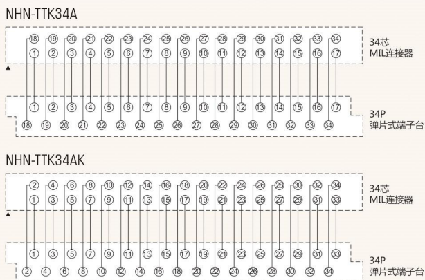
配线图 Wiring Diagram
