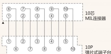
配线图 Wiring Diagram
