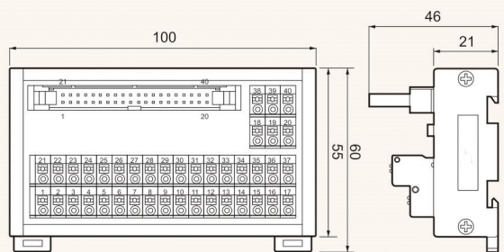
外形尺寸图 Dimensions
