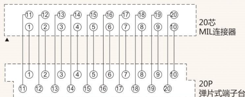
配线图 Wiring Diagram
