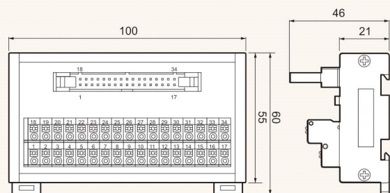
外形尺寸图 Dimensions
