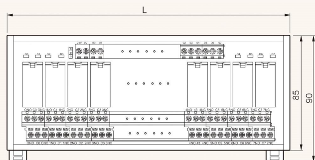
配线图 Wiring Diagram
